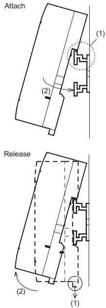
Figure2. Installation Diagrams Installations-Skizze Diagrammes d'installation Diagramma di installazione Esquemas de instalación Installationritningar
